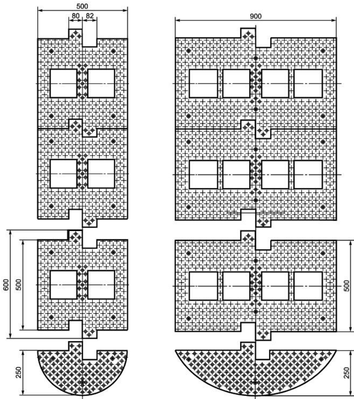
Рисунок Б.1 - Пример конструкции типовых ИНС
