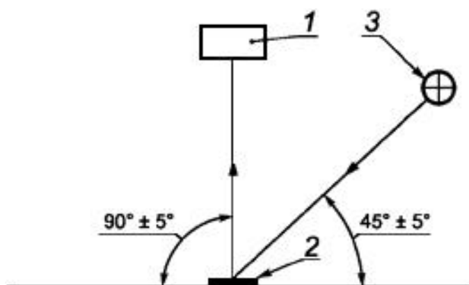
Рисунок 4 - Условия измерения координат цветности и коэффициента яркости
